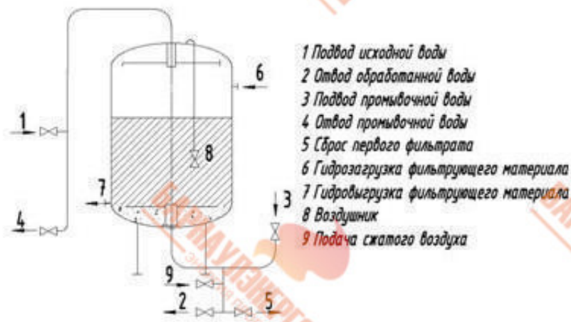
Схема работы фильтра
